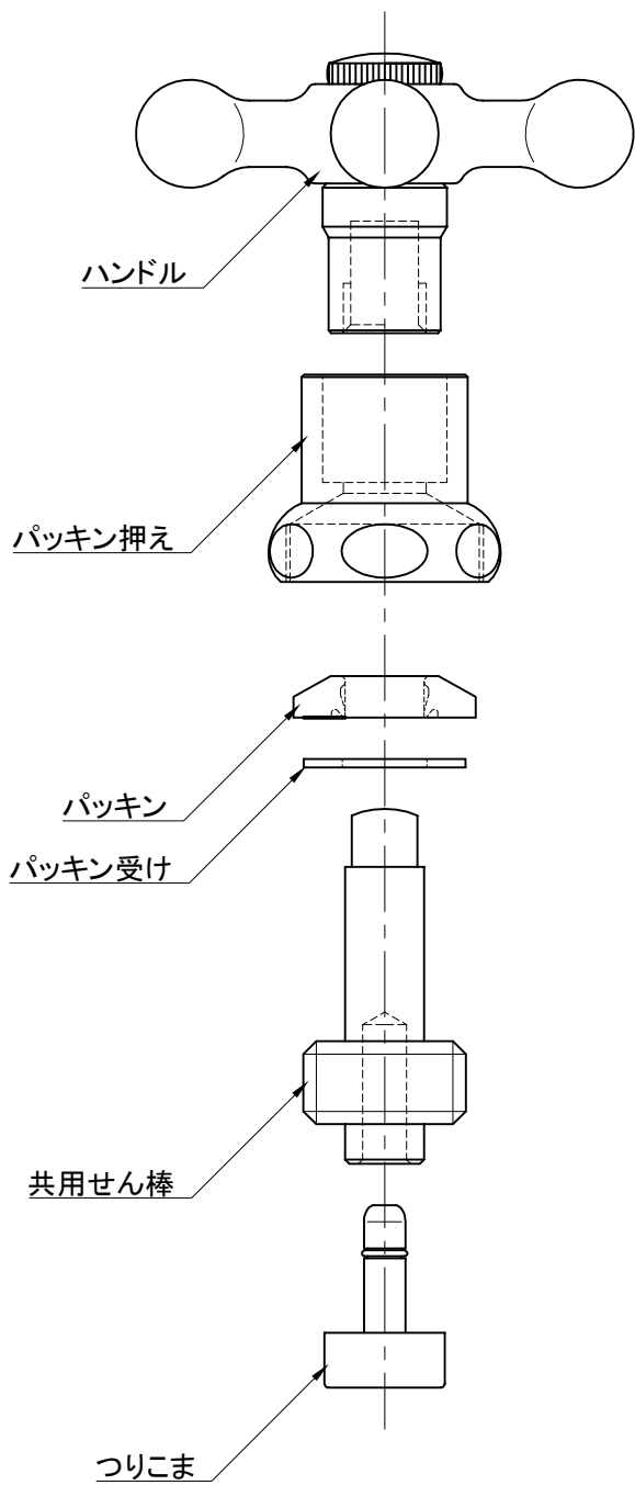
部品構成
