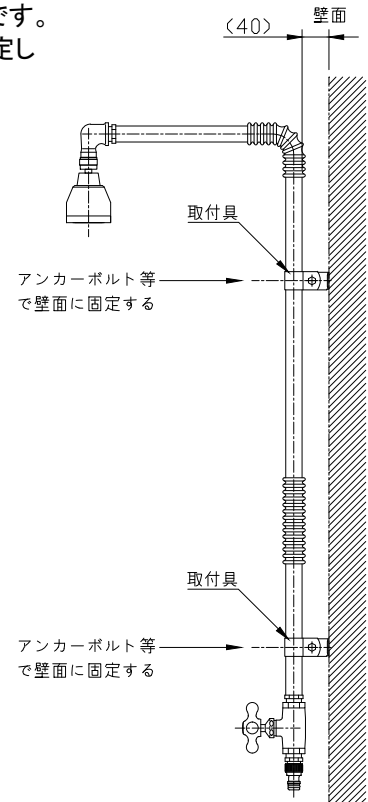
参考取付図
